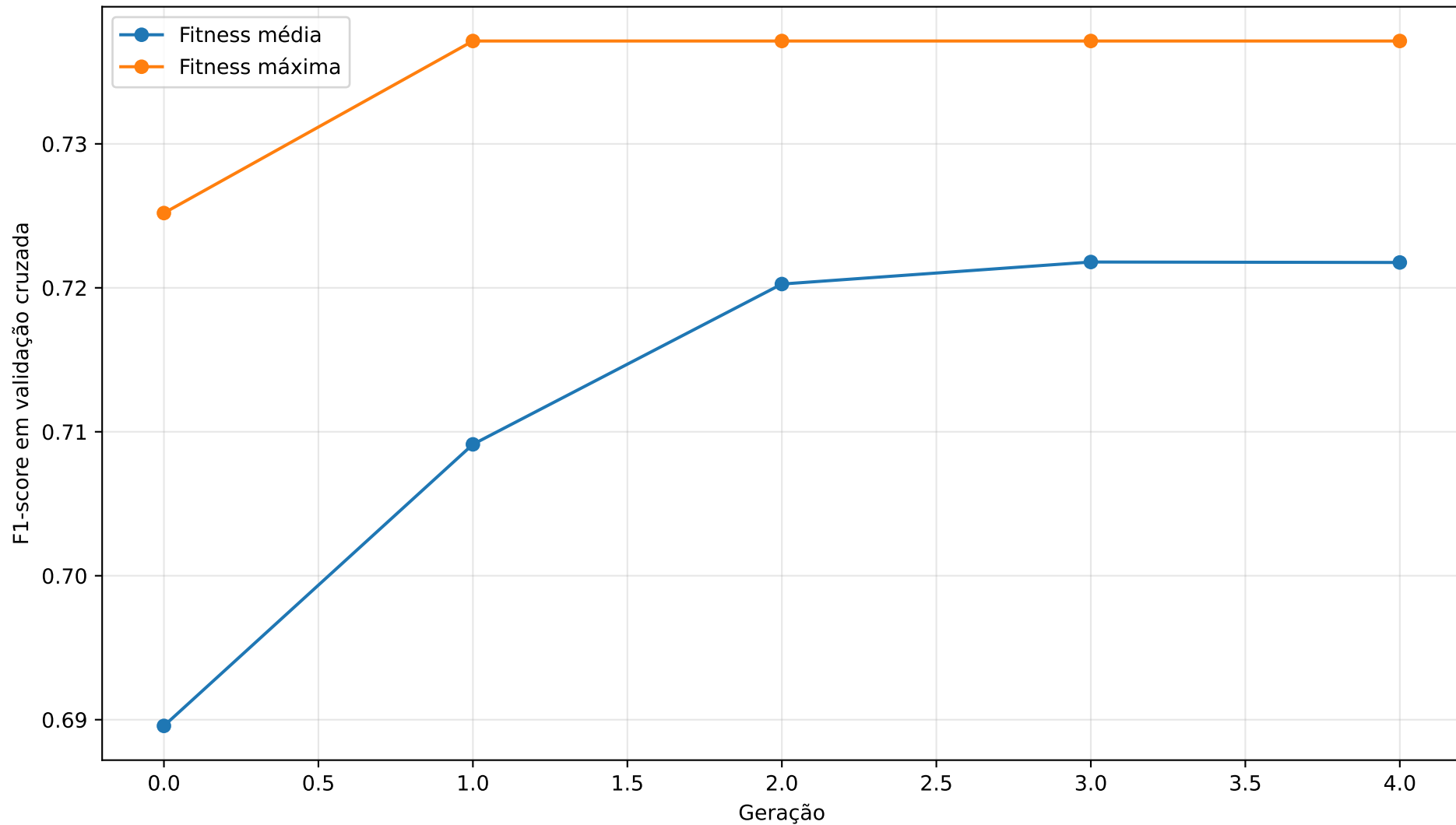
Convergência do GA de Hiperparâmetros
